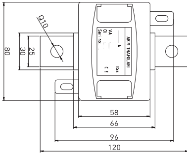
Teknik Resim
