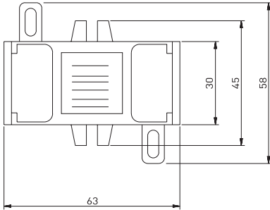
Teknik Resim
